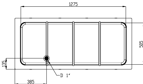
Boven aanzicht
